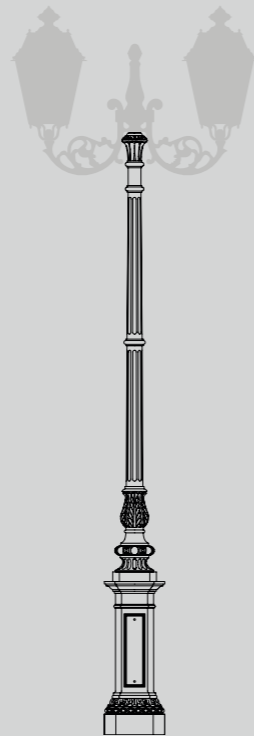
Castore palo h 4 m Lanterna Light 600
