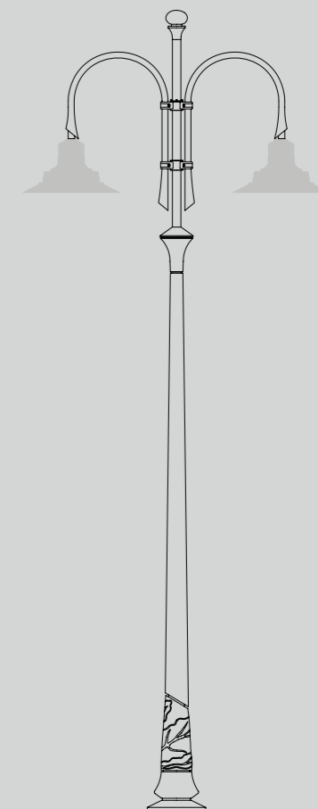
Alcor palo con bracci h 4, 5 e 6 m Lanterna Light 21
