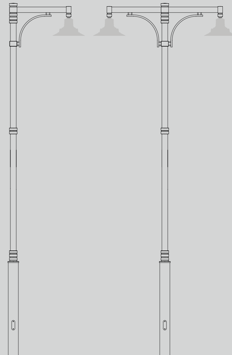
Mizar palo con braccio h 6, 7 e 8 m Lanterna Light 22
