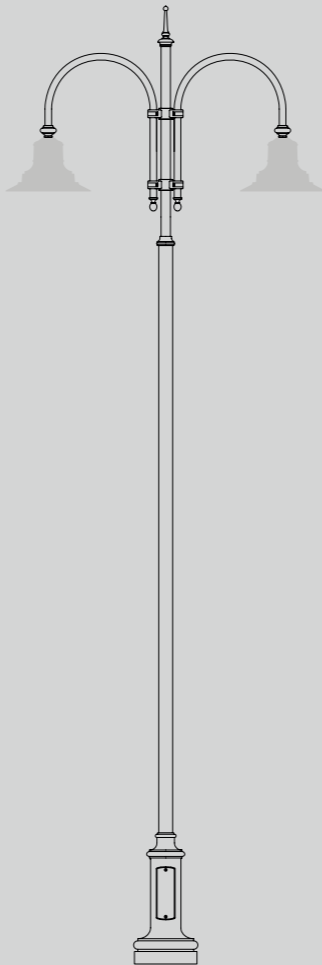
Kuma palo con bracci h 4 e 5 m Lanterna Light 21
