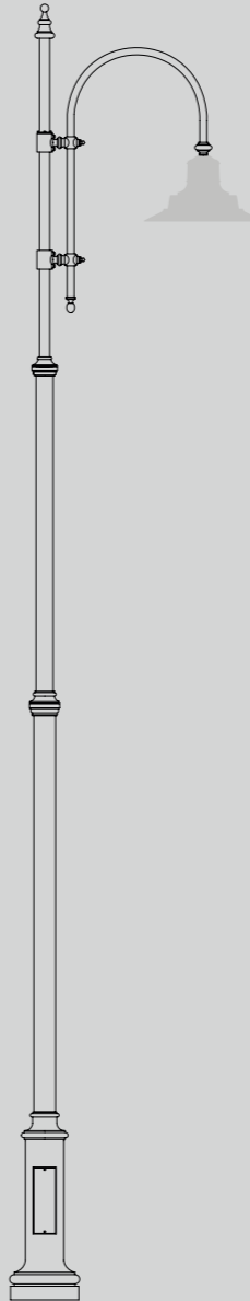
Kuma palo con braccio h 6 e 7 m Lanterna Light 22
