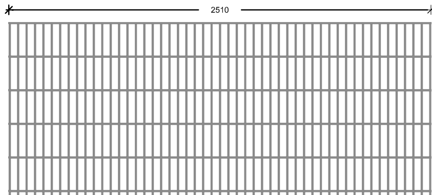
Rete metallica
