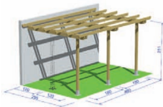
PERGOLA LUNA ADDOSSATA LUNA MOUNT. PERGOLA
