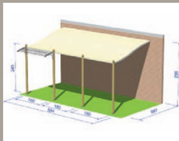
PERGOLA MOTUS ADD. COP. PVC MOTUS MOUNT. PERGOLA PVC COV.
