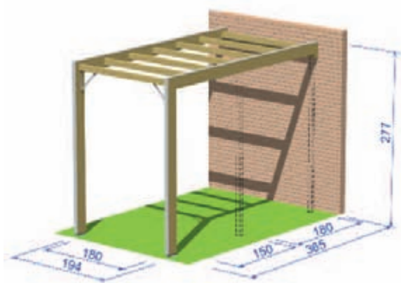
PERGOLA SPAZIO ADDOSSATA SPAZIO MOUNTED PERGOLA
