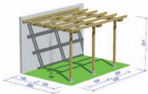
PERGOLA LUNA ADDOSSATA LUNA MOUNT. PERGOLA
